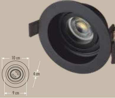
CT-5020 PARS (3'LÜ SİYAH)
