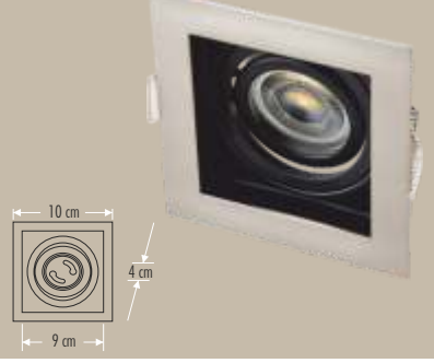
CT-5223 PARS (SİYAH)
