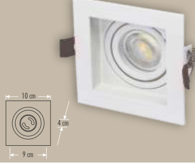
CT-5222 PARS (BEYAZ-SİYAH)
